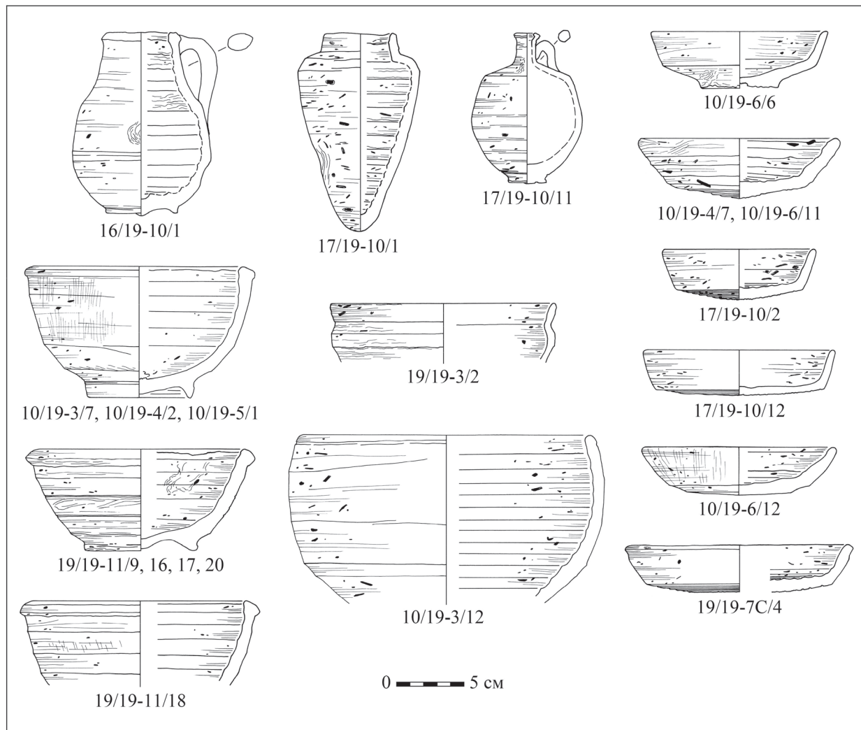
Илл. 6. Керамика Позднего периода из шахт 3, 4, 5, 6, 7, 11 и ниши 10 гробницы Перинеджу в Гизе (рис. автора)
