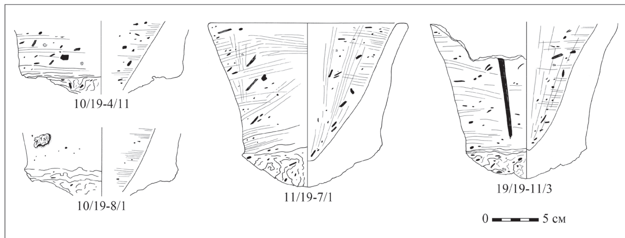
Илл. 4. Конические хлебные формы времени V–VI династии из шахт 4, 7, 8 и 11 гробницы Перинеджу в Гизе (рис. автора)
